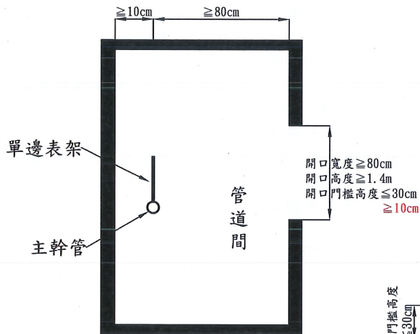
俯視圖
