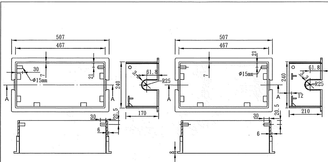
小型水表箱(口徑20~25mm) 單位：mm
