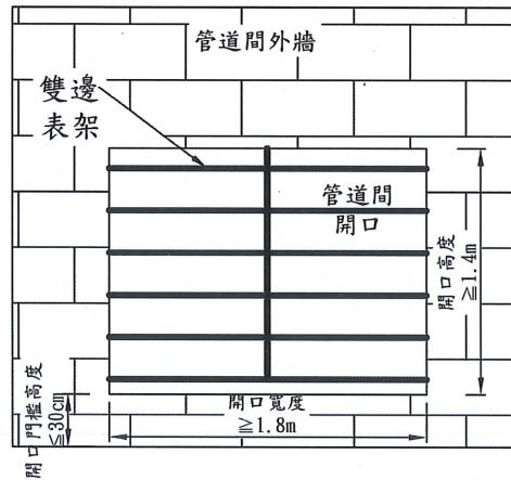
管道間開口正視圖
