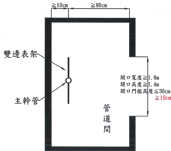
俯視圖
