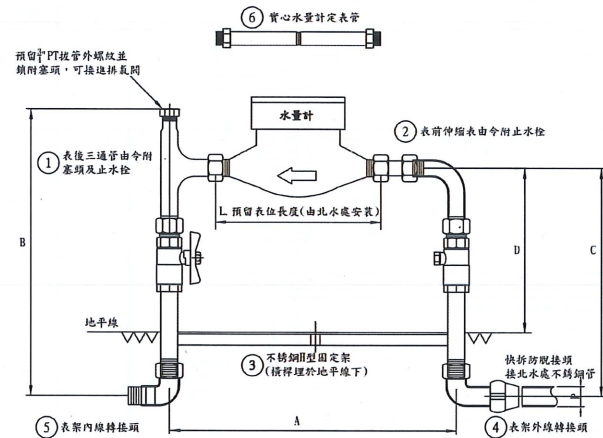
地上式中、小表表位架示意圖
